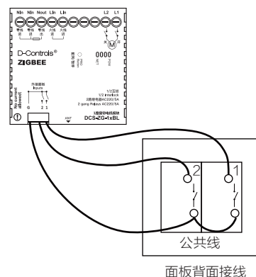
面板背面接线
