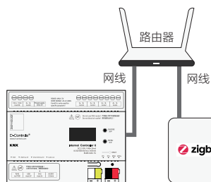
KNX中控主机 型号：IC6
