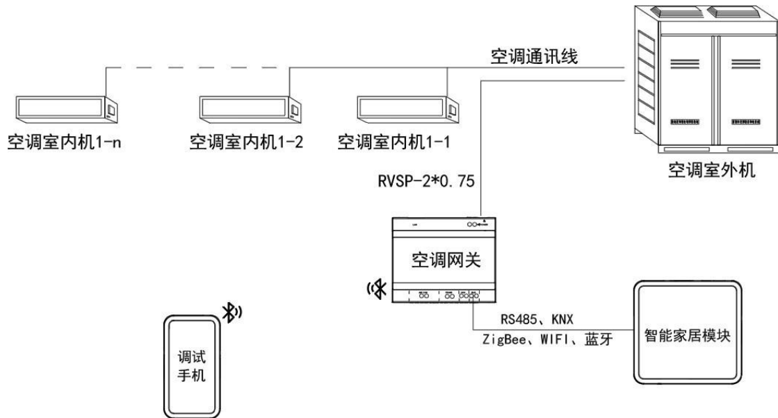
图 3 系统接线图
