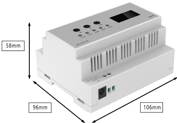
图1 外观及尺寸设备组件图
