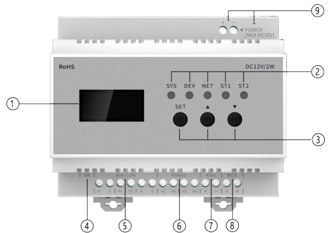
图2 端子及指示说明
